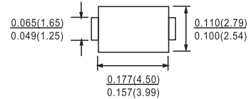
DO-214AC(SMA)
