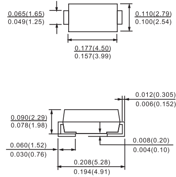
DO-214AC(SMA)
